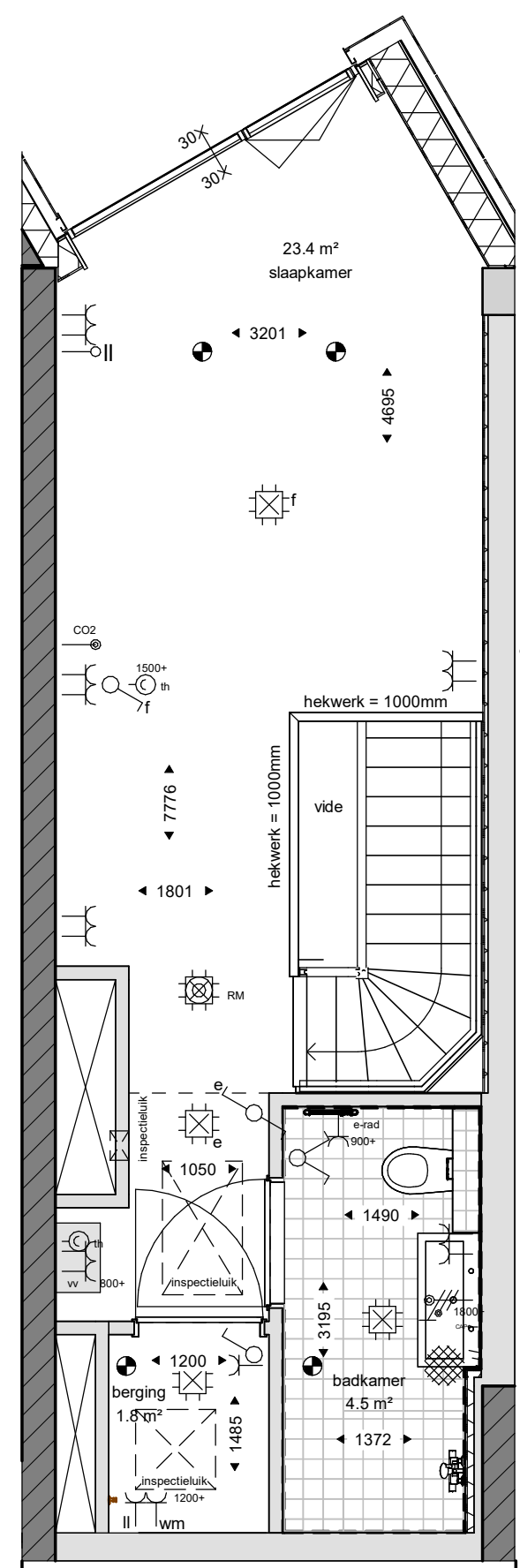
eerste verdieping
